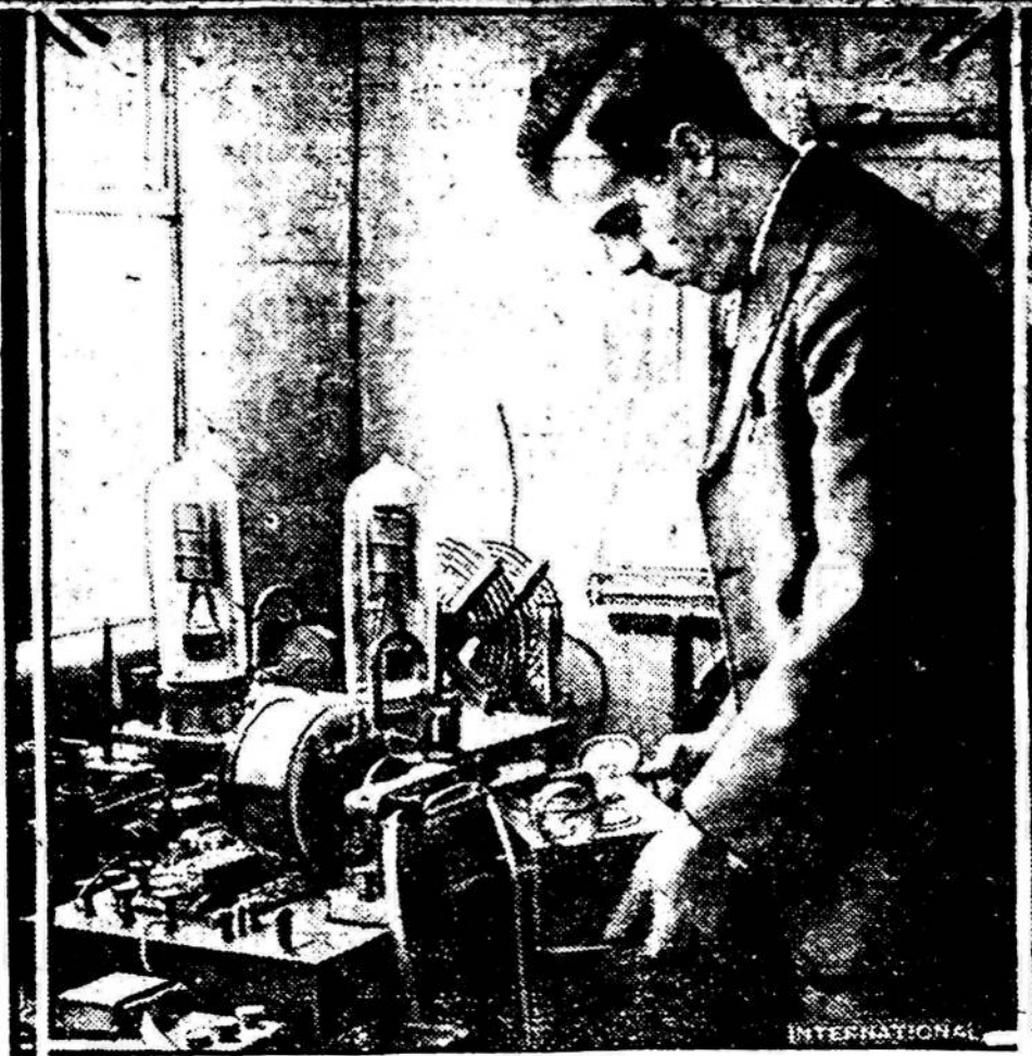
Čia parodoma bevielio telegrafo stoties aparatas Richmond Hill, L. I. Tas aparatas toks stiprus, kad susineša su orlaiviais ir galės susinešti su orlaiviais, lėksiančiais į šiaurinį asi-galį.
