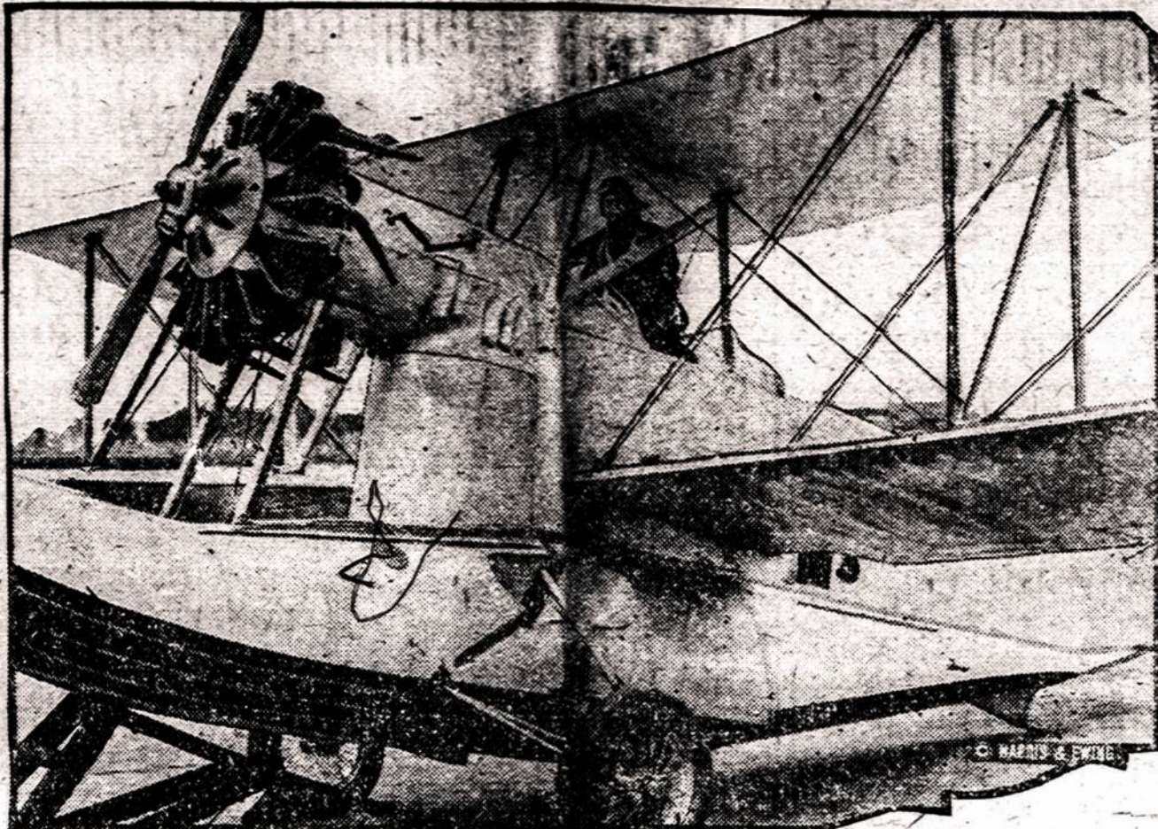
Čia parodo gal būt pirmą orlaivį, kuris gali plaukti vandeniui ir lėkti oru ir su mo- toro šildytuvu, ką tik atvežtas į jūrėivijos oro stotį Washingtone, kur jį nuodugnai per- žiūrėjo. Šio orlaiviu lekiant gal būt bus mažiau nelaimių ant jurių.
