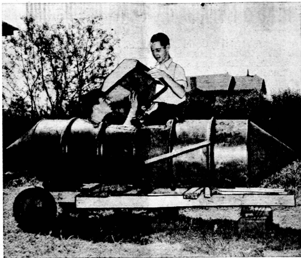
ISRADEJAI — Jimmy Dale, kairė, ir Emmitt Kelly pradėjo dar peraitą pavasarį statyti nardomąjį šalmą savo namuose Dallas, Texas. Jų darbas davė vaisių, nes pripažinta, kad tas jų nardomasis šalmas yra geras vieno žmogaus submarinas. Jis daro keturias mylias per valandą po vandeniui.
