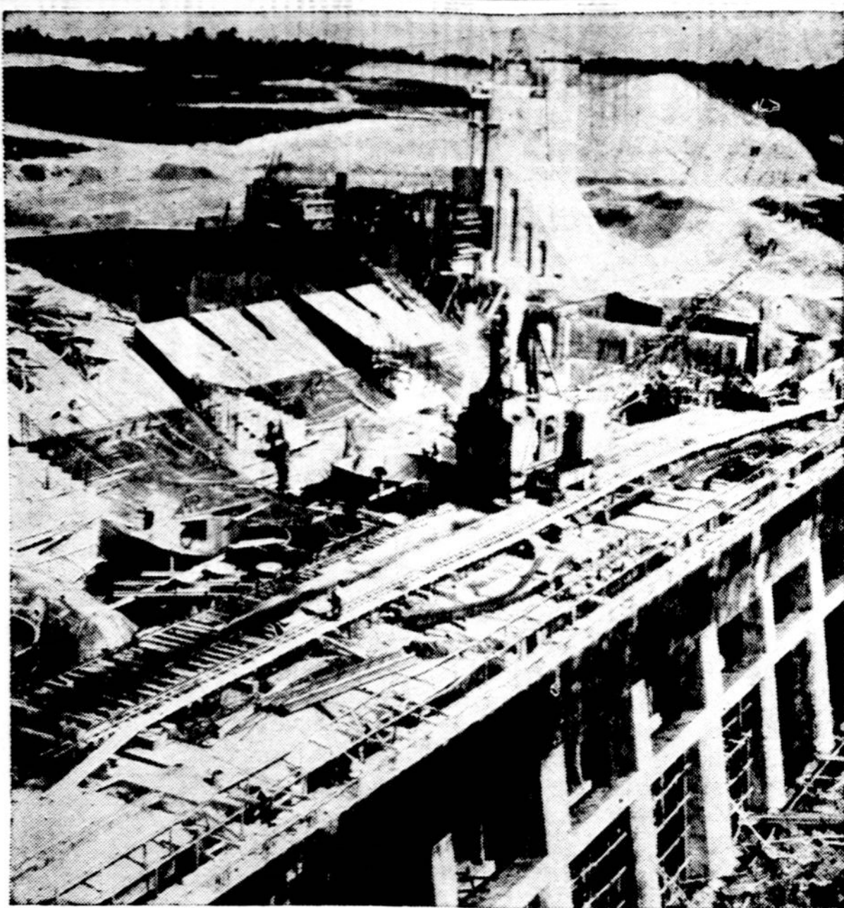
Čia matome milžinišką Santee-Cooper hidro-elektros ir navigacijos projektą, kuris skubiai statomas, kaip vienas iš apsigynimo darbų. Šis milžiniškas projek- tas statomas Charleston, S. C.
