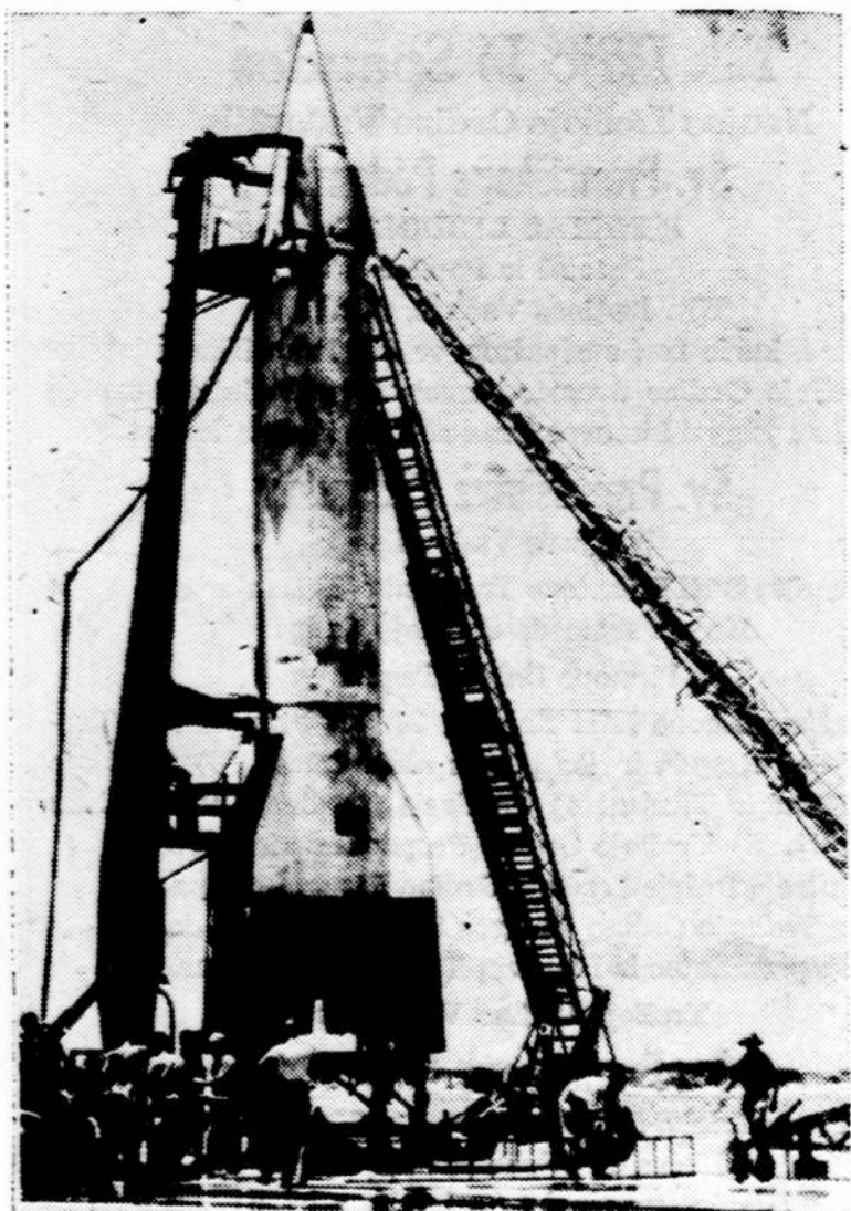
Paveikslas šios milžiniškos raketos buvo pagautas tik prieš pat jos iššovimą White Sands Proving Grounds, N. M. Buvo manyta, kad ši V-2 raketa pasieks 100 mylių aukščio, bet pasiekė tik 75 mylias.
