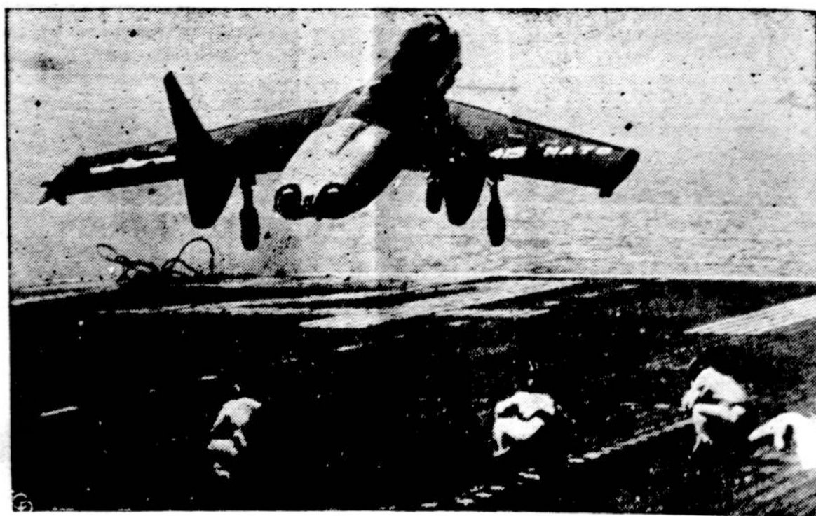
Sprausminis lėktuvas pakyla nuo lėktuvnešio U.S.S. Midway. Lėktuvas sveria 20.000 svarų. Jo ilgis per sparnus 40 pėdų. I orą jis nusiviedžiamas stipraus prietaiso (katapulto).
