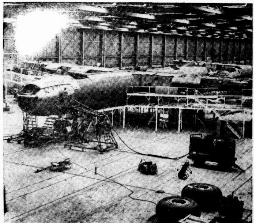
B 36 bombonešų dirbtuvė Fort Worth, Tex., perdirbama atominė energija varomiems lėktuvams gaminti. Manoma, kad atominis lėktuvas bus brangesnis net už atominį povandeninį laivą, kurio statybai jau išleista 40 milijonų dolerių.
