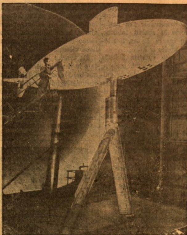
Tai modelis pasaulyje greičiausio povandeninio laivo, dabar bandomo vėjo tunelyje surasti geriausius valdymo būdus.
