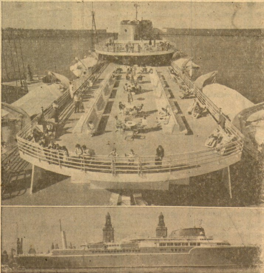
Didžiaisiais ežerais keleivius vežioti paleistas toks $8,000,000 vertės laivas, turįs visus modernius patogumus. Nuo 1957 metų jis pastoviai kursuos tarp Clevelando ir Detroito.
