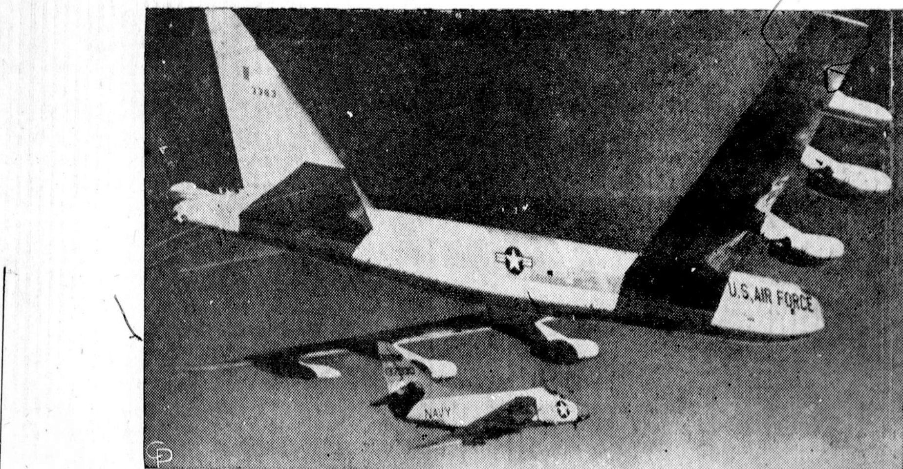
Tai didžiausias ir mažiausias JAV sprausminis kovos lėktuvas. Didysis — B-52 yra 156½ pėdų ilgio, 185 pėdų sparnų pločio ir sveria 450,000 svarų. Mažasis — A4D tik 39 pėdų ilgio, 27½ sparnų pločio ir sveria 15,000 svarų.
