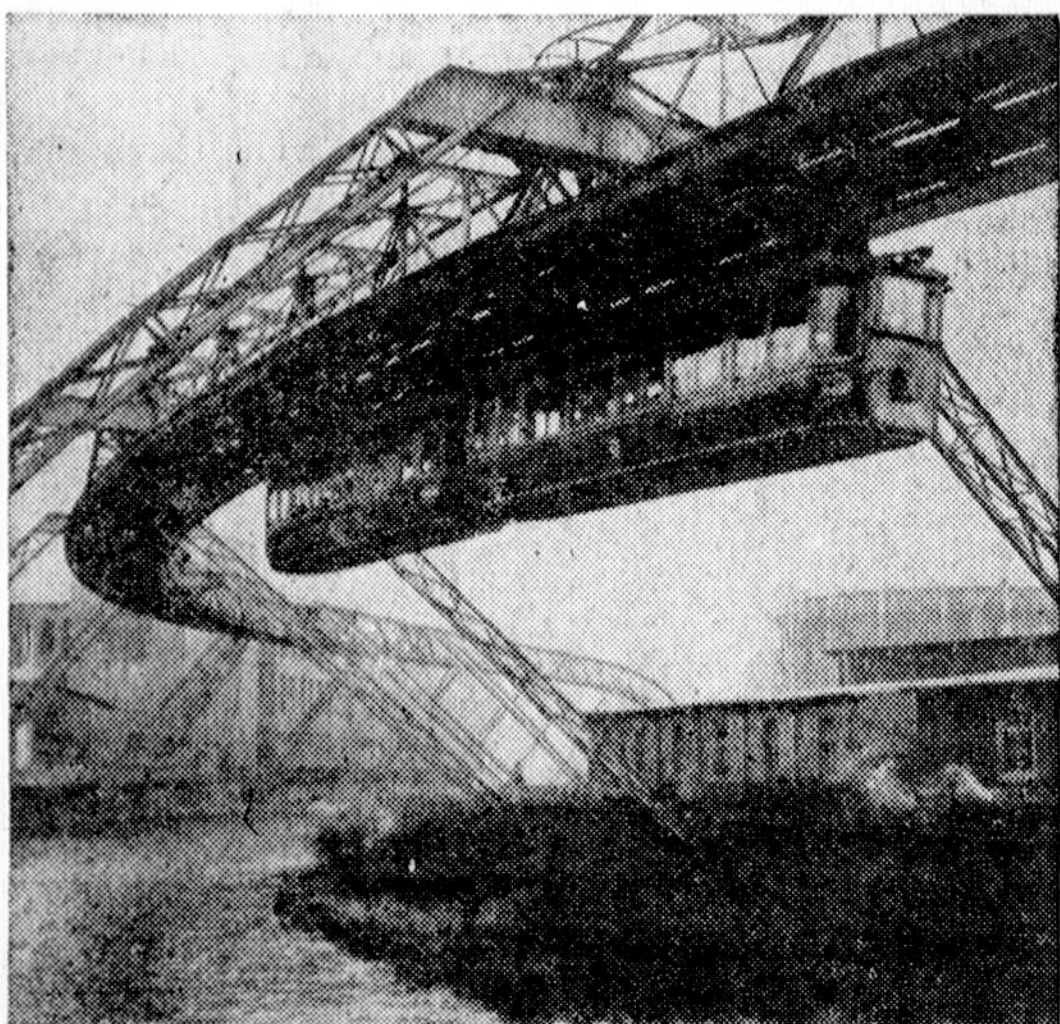
Kada JAV miestai kaskart vis labiau užkemsami automobiliais, susisiekimo specialistų akys krypta į tokį kabančią traukinį, kuris jau 50 m. sukaktį švenčia. Tai Wuppertalio, Vakarų Vokietijos, kabančias traukiny.
