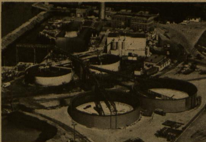
Water Treatment Plant at Republic's karšto ir šalto metodo plieno apdirbimo vietovėje atnaujinama daugiau kaip 100 milijonų galionų vandens kasdien. Originali kaina $18 milijonų. Papildomas vandens išvalymas: $6 milijonai.
