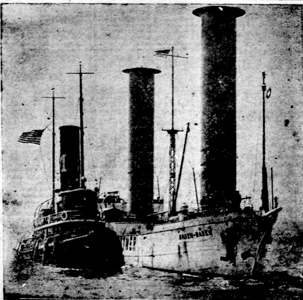
Naujai išrastas vokiečių rotorinis laivas, kuris smarkiai plaukioja be žėglių ir be mo- toro. Jį lydi į prielauką Amerikos laivelis.
