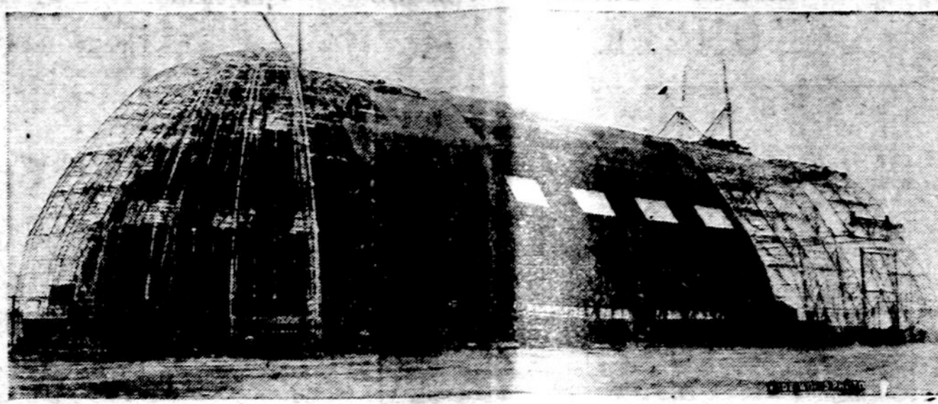
Šitas milžiniškas angaras yra statomas Akrono mieste, Ohio valstijoje, kur bus daromi milžiniški dirizabliai, dvigubai didesni už vokiečių "Grafe Zeppelina", kuris neseniai apiekė aplink visą žemės kamuolį.
