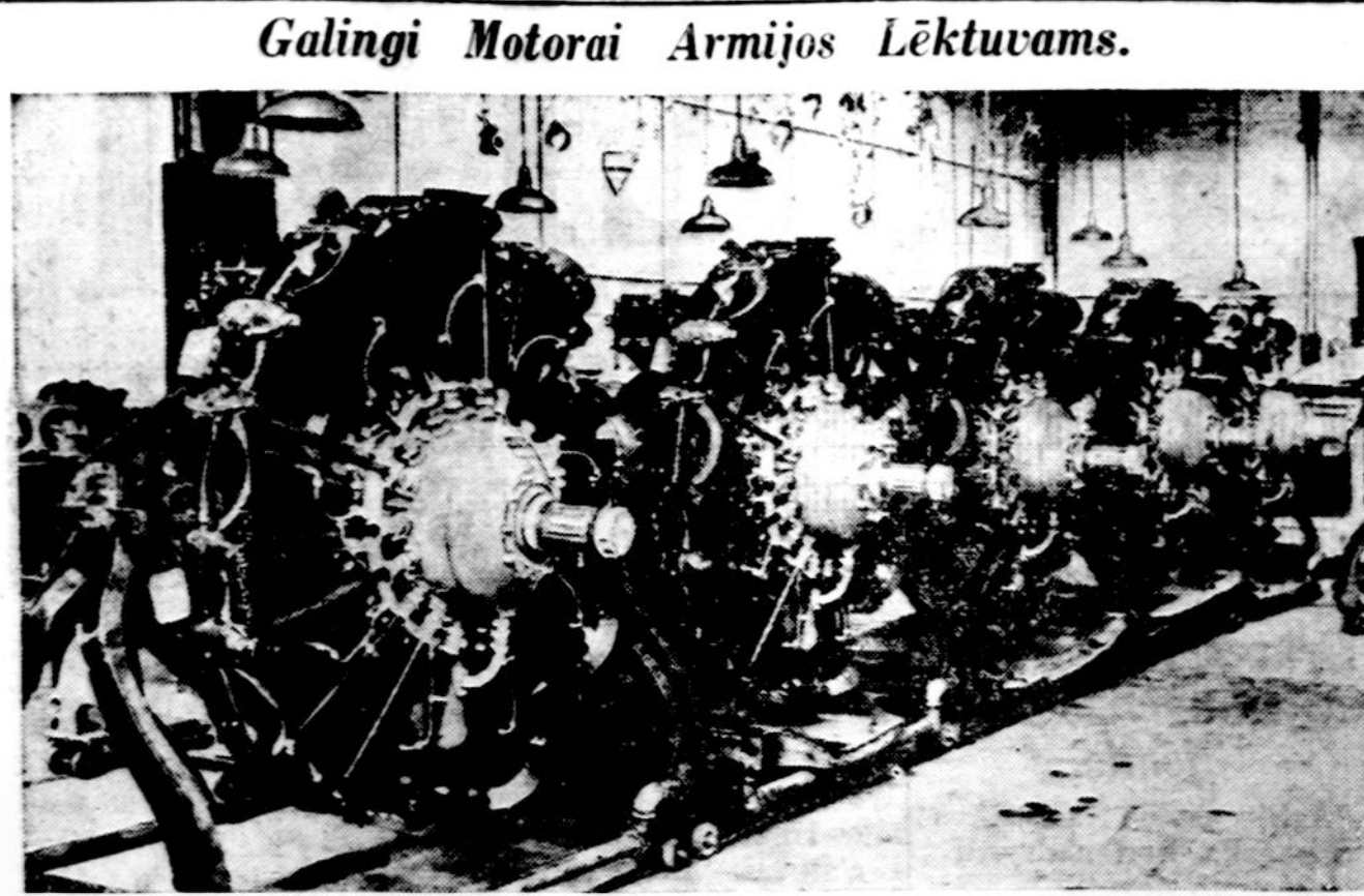
Stai, kaip išrodo "Cyclone" tipo varikliai armijos orlaiviams. Washingtono valdžia užsakė 150 šitokių motorų iš Wright Aeronautical korporacijos. Jie turi po 1,000 arklių jėgos pakilant nuo žemės. Jie buvo bandomi ir tobulinami per 10 metų, pakol galų gale tapo pripažinti kaip tinkamiausi varikliai karo lėktuvams. Nuo kitų motorų jie skiriasi tuo, kad labai greitai pakla- la su dideliu kroviniu ir išvysto labai didelį greitumą pakilę didelėn aukštumon. Už 150 moto- rų valdžia moka $1,327,190.
