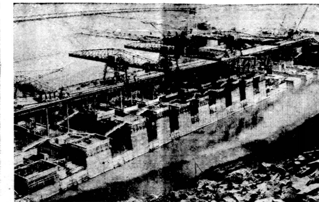
Čia vaizdelis parodo paruošiamuosius darbus Grand Coulee užtvankai, kuri bus pastatyta per Columbijos upę. Parodyta čia siena yra statoma visų pirmą upės vagai nukreipti į šalį, kad paskui galima būtų statyti pačią užtvanką. Užtvankos upės vanduo bus pakinkytas elektros energijai gaminti. Ši užtvanką bus didžiausia visame pasauly. Ją stato federalinė valdžia, kad davus bedarbiams uždarbio ir kad paskui kraštui būtų iš to naudos. Columbijos upę pradedada Kanadoj, paskui teka Washingtono ir Oregono valstijų rubežium ir įteka į Ramųjį Vandenyną.
