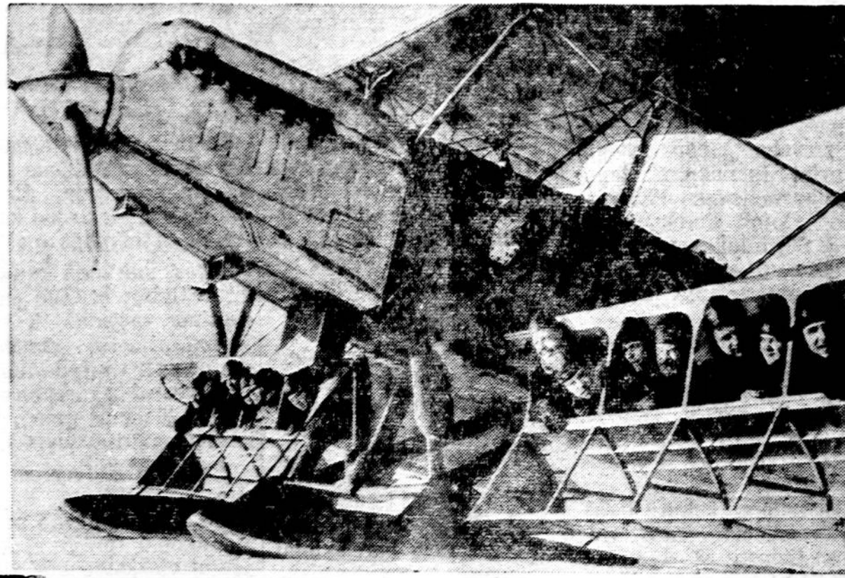
Čia parodytas naujos konstrukcijos Sovietų armijos lėktuvas, kuris sėdines žmonėms turi įtaisytas po sparnais. Jis neša 16 žmonių.
