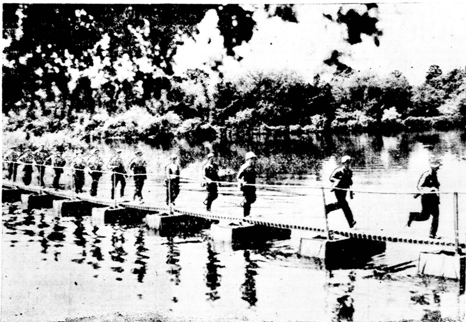
Dabar Jungtinės Valstijos daromi karo pratimai arba manevrai, kuriuose bandomos Europos karo naujybės. Šiame vaizdely ant greitųjų inžinierių nutiestas tiltas per upę. Jis laikosi ant laivelų, kurie yra įkabinti į pės dug- nā tam tikrais įkrais. Šis tiltas buvo nutiestas pereitą savaitę ties Norwoodo, New Yorko valstijoje.
