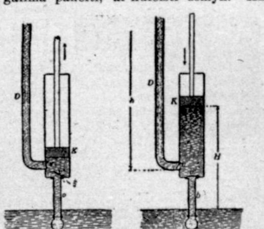
Darbas keliančios-spaudžiančios vandenį pompos.
