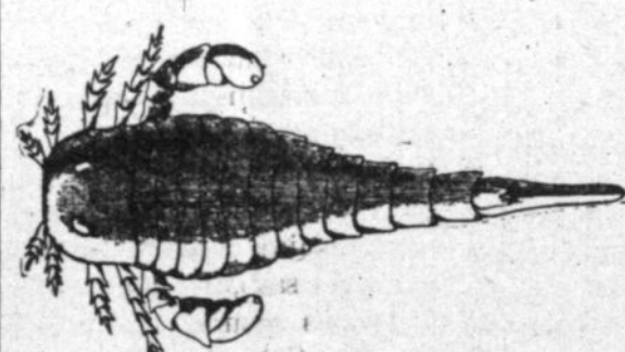
Vėžys iš siluriskos formacijos. Paveikslas persiūto tikro gyvūno didumą. Pagal Frana.
