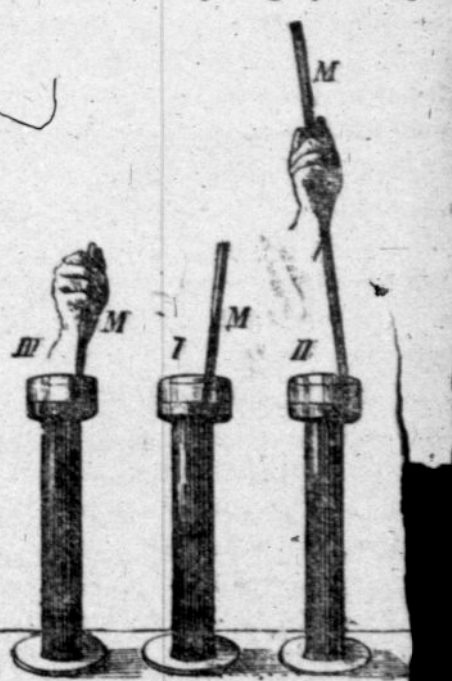
Vienodas daugumas/gazo nevienodai užima ruimą, tas paeina nuo spaudimo ir temperatūros.
