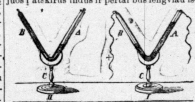
Surinkimas gazų padalinant vandenį elektrika.
