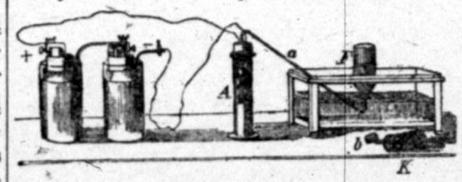
Surinkimas gazų, besidarančių padalinant vandenį elektrika.
