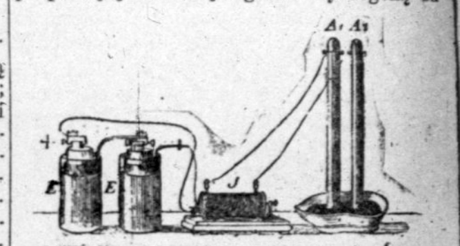
Padalinimas vandens į sudėti- nius pagalba elektrikos.
