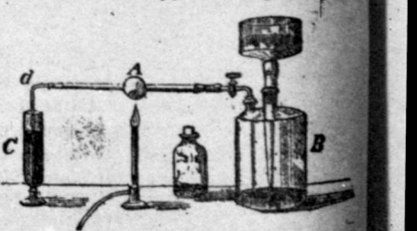
Besidarymas angliarugšties iš angliadario ir oxygeno.
