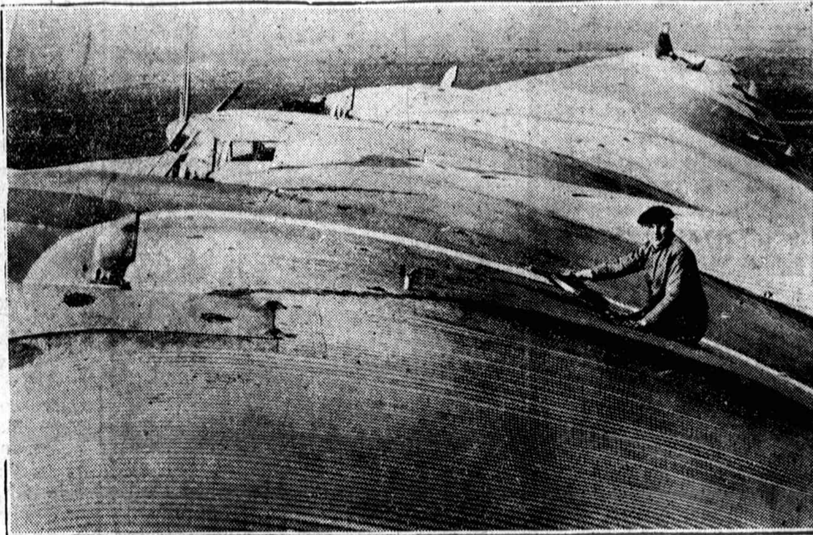
Didžiausias pasauly Junkerio aeroplanas—G-38, kuris dabar yra bandomas. Vaizdas nuo aeroplanų sparnų, 147 pėdas ilgumo. Aeroplanas varomas keturių inžinų, bendrai 2.400 arklių jėgos. Pasazieriai bus gabenami sparnuose.
