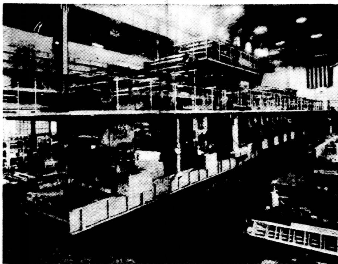
Pirmas po karo padirbtas rotary web press, laikraščiams ir knygoms spausdinti mašina. Ją padirbo R. Hae ir Co., dėl St. Louis Post-Dispatch.
