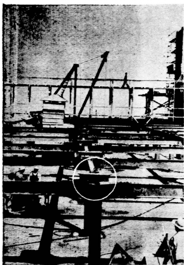
Naujos rūšies statyba Los Angeles statytojų turės namų fundamente 65 setus "roller bearing", kurie laike žemės drejbėjimo leis namui pasislinkti šešius colius. Vaizdas parodo tos statybos planą ir apskritime vieną iš minimų "roller bearing".
