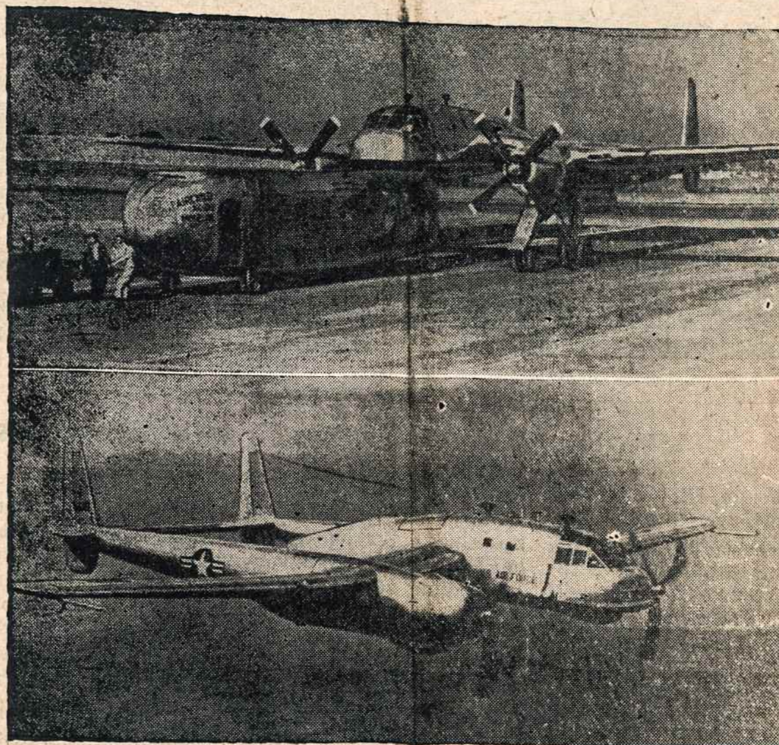
Bandomas naujas transportinis lėktuvas KC-120. Viršuje matome dvi jo dalis. Vienna, vidurinė, gali būti ištraukta, prikrauta važmos ir vėl pastumta po lėktuvu, kuris ją perkelia ir nusiveža, kur reikia. Apačioje lėktuvas grįžta be krovinių. Jam nereikia laukti, kol iškraus ar pakraus.
