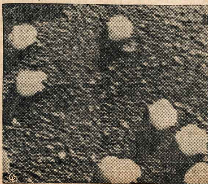
AZIJOS GRIPŲ bacilos, padidintos 220,000 kartų
