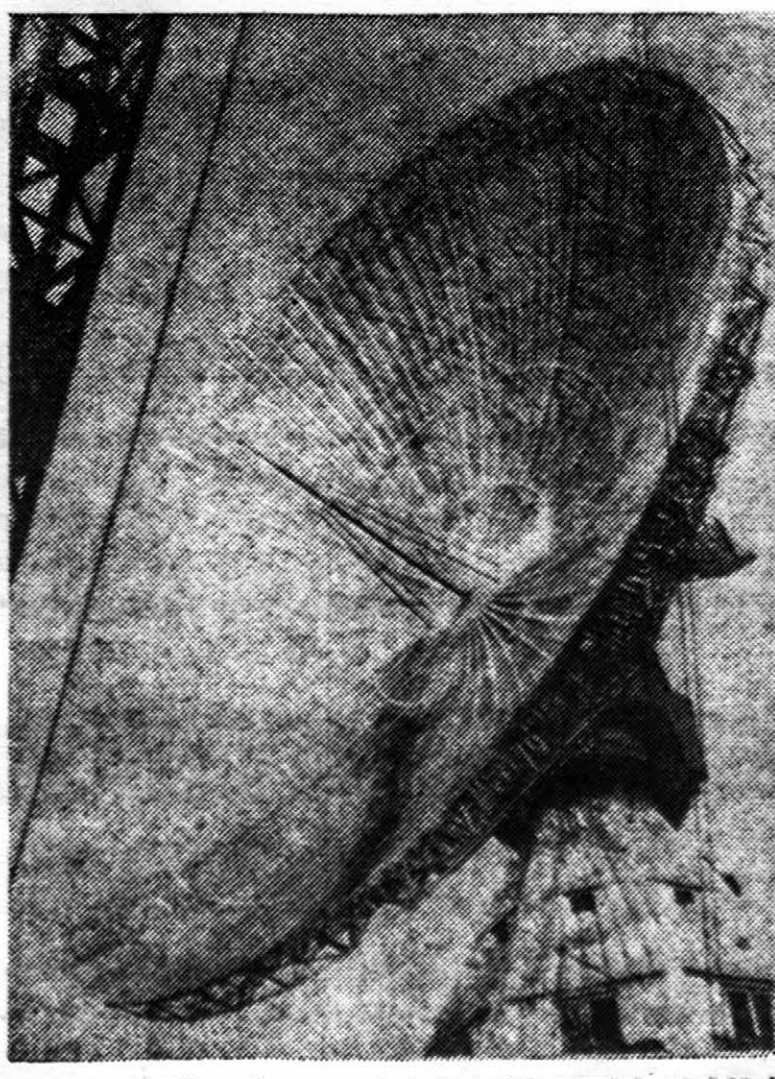
Radio teleskopas, didžiausias pasaulyje tos rūšies erdvių stebėtojas, baigtas statyti Vakarų Vokietijoje Eifelio kalnuose.
