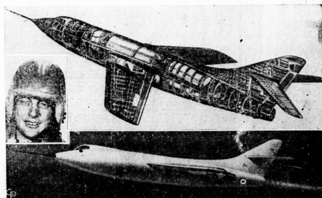
Amerikos laivyno raketinis lėktuvas D-558-2, kuriuo lakūnas Bill Bridgemanas iškilo iki 78,000 pėdų aukščio ir pasiekė greitį apie 1,300 mylių per valandą. Lėktuvas paleistas ne nuo žemės, bet nuo kito lėktuvo — bombonešio, kuris jį iškėlė prieš paleidžiant į 35,000 pėdų aukštį. Paveikslė matoma lėktuvo išvaizda, jo skersinis pjūvis ir lakūnas Bridgemanas.
