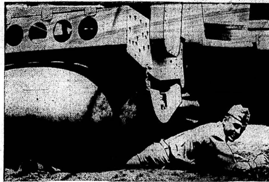
Detroito arsenalo inžinieriai išrado mašiną, kuri lengvai važiuos per pelkes ar 17 pėdų sniegą. Pavadinta Relitron. Ji turi nylo no maišus vietoj ratų. Maišai upadūziasi prie grandinėmis varomų volų. Kai volai juda, jie suka maišus ir mašina važiuoja.
