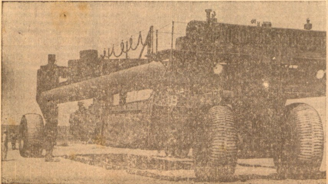
Tai ne pabaia, bet laivų kėlimo mašina. Ji lengvai pakelia 67 tonų laivą iš vandens į krantą.
