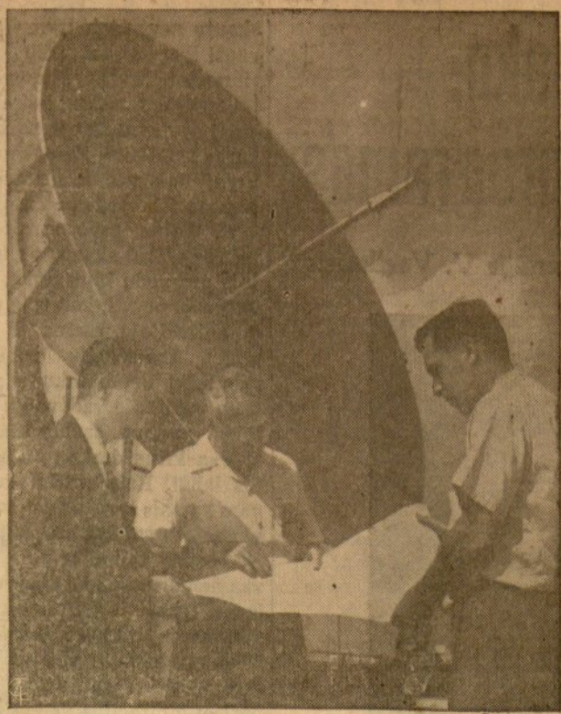
Trys astronomai, kurie moderniais prietaisais tyrinėja Venerą, tikina, kad ten esanti 220 laipsnių temperatūra. Jie darbiu naudoja 50 pėdų ilgio teleskopą.
