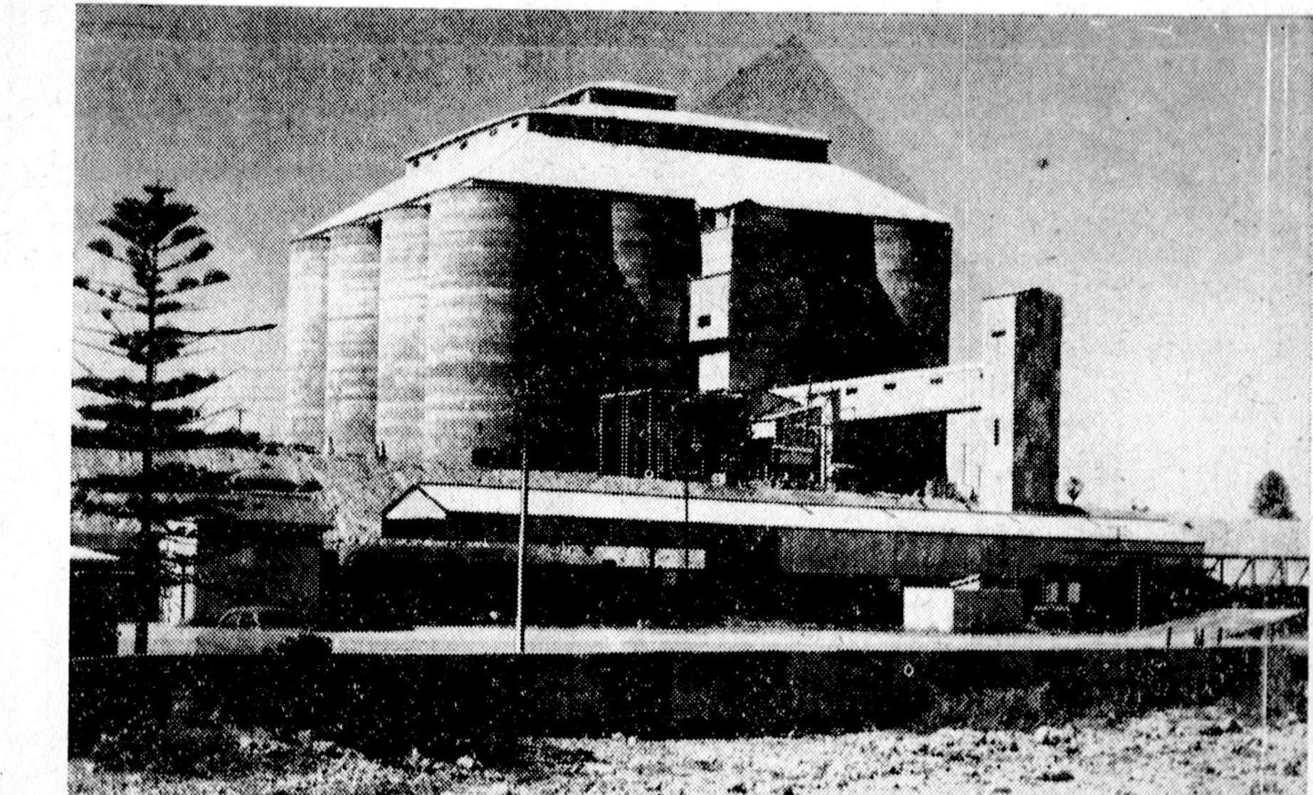
Didžiulis javų elevatorius Adelaidėje, Australijoje, kurio statymą prižiūrėjo lietuvis inžinierius A. Pacevičius. Tai didžiausias tos rūšies pastatas Australijoje, talpinąs 1,500,000 bušelių javų. Plačiau skaityk J. Bačiūno kelionės aprašymus.
