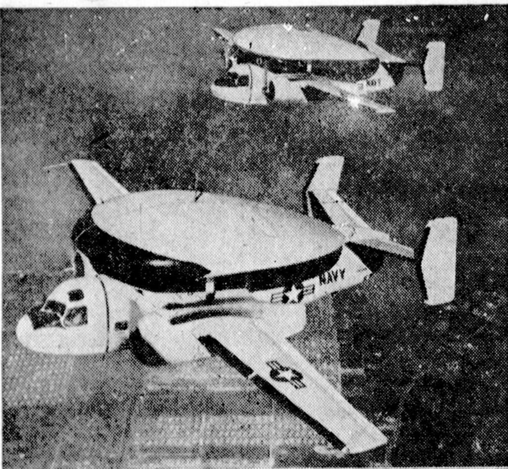
Pirmas modelis JAV laivyno Grumman WF2 radarinio lėktuvo, kuris skrenda virš New Yorko. Didelis radaras viršų sudaro skraidančios lėkštės vaizdą.
