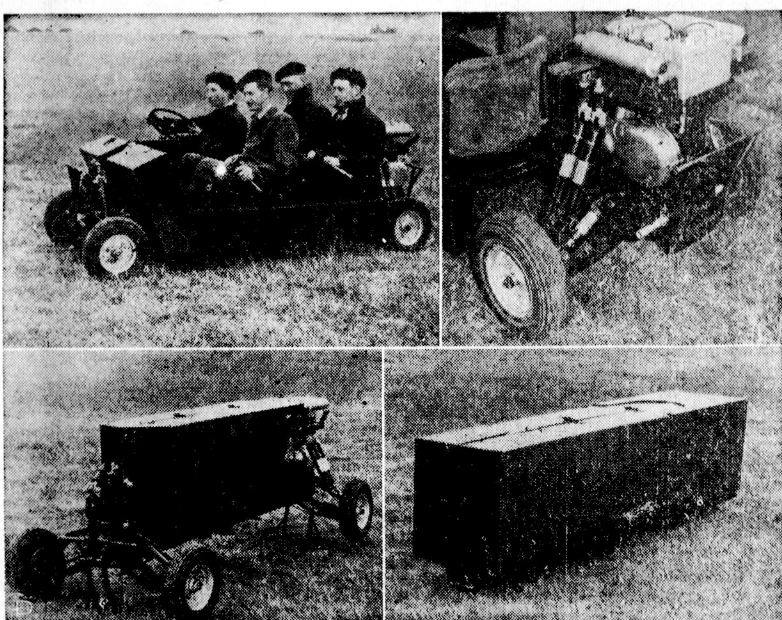
Ši nauja, anglų sukonstruota mašina, su savim nešasi ir garažą. Ji sveria tik 700 svarų, o suklankstyta užima labai mažą vietos. Ji tai pat lengvai nuleidžiama parašutu iš lėktuvo.
