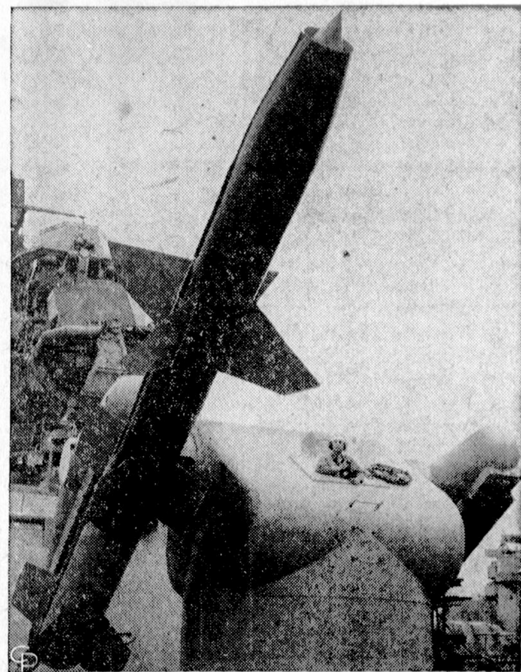
Galveston kreiseris, pirmasis iš JAV laivų, buvo apginkluotas Bendix Talos 3000 svarų spausminėmis raketomis. Jos skirtos naikinti priešų lėktuvus, esančius iki 65 mylių atstume ir dideliuose aukščiuose.
