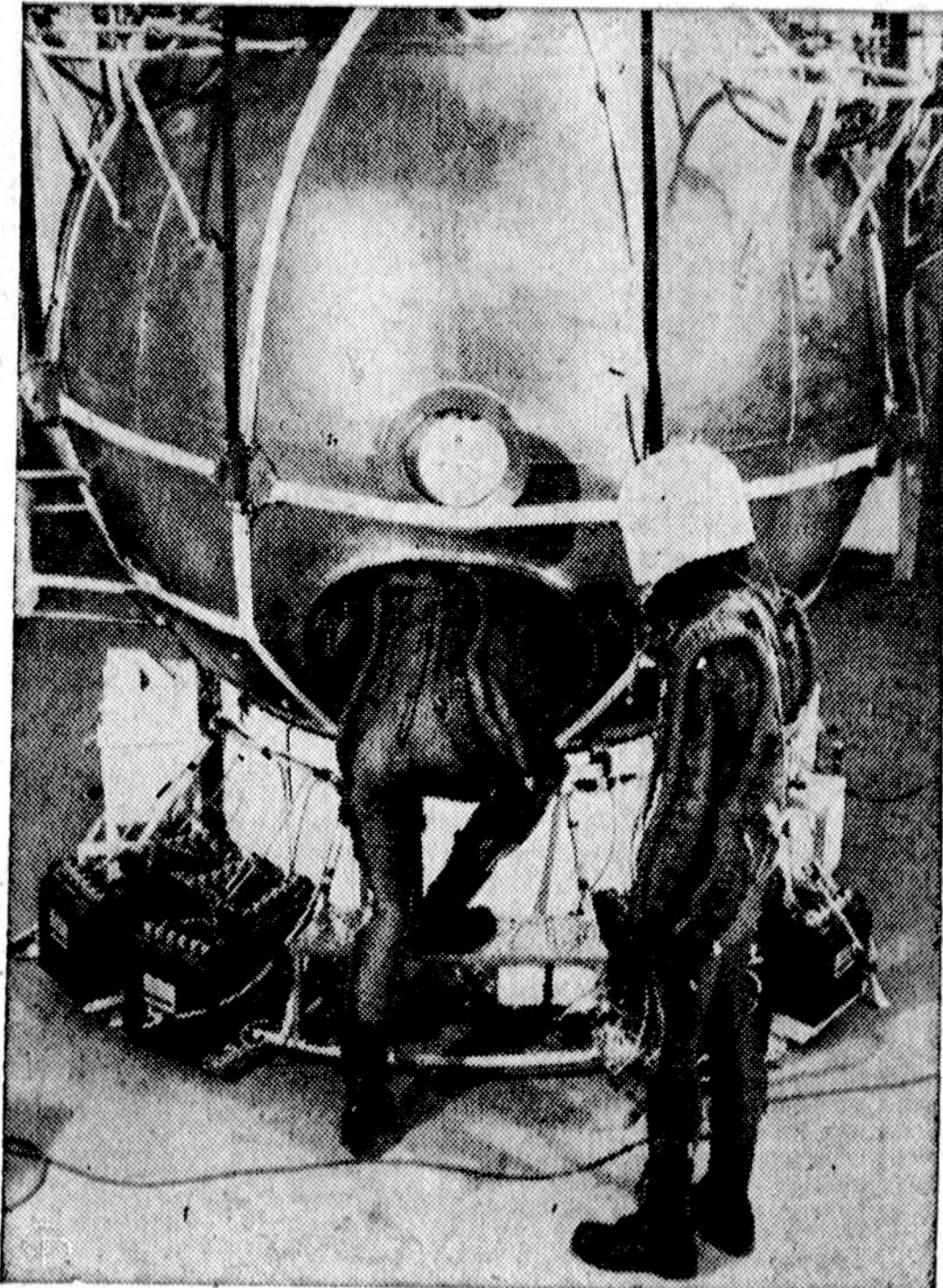
JAV mokslininkai L. Lewis ir M. Ross balionu pakilo į 80,000 pėdų aukštį tirti kosminio spinduliavimo. Kildami jie pasieė apie 5,000 vabzdžių, įskaitant namines muses ir bites, kad nustatytų to spinduliavimo įtaką vaisingumui.
