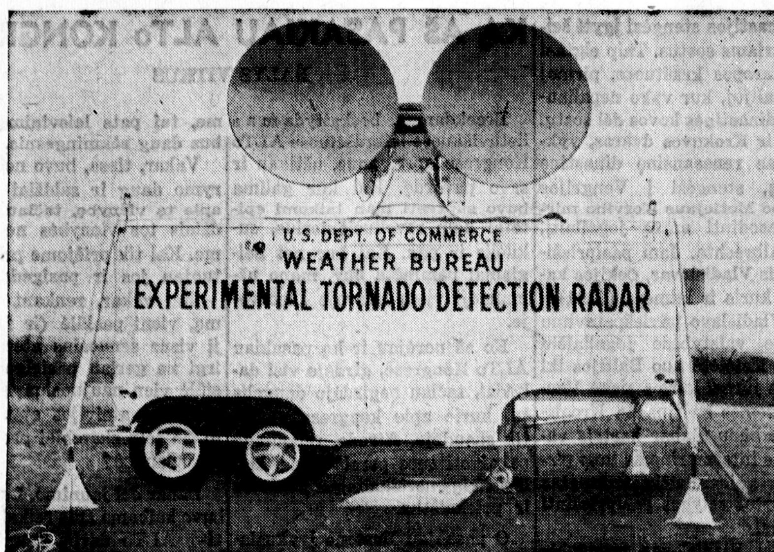
Wichitoje, Kansas, bandomi naujos rūšies radaro įrenginiai vėjo stiprumui matuoti. Tikima, jog šie įrenginiai pagelbės iš anksto įspėti gyventojus apie artėjančias audras.
