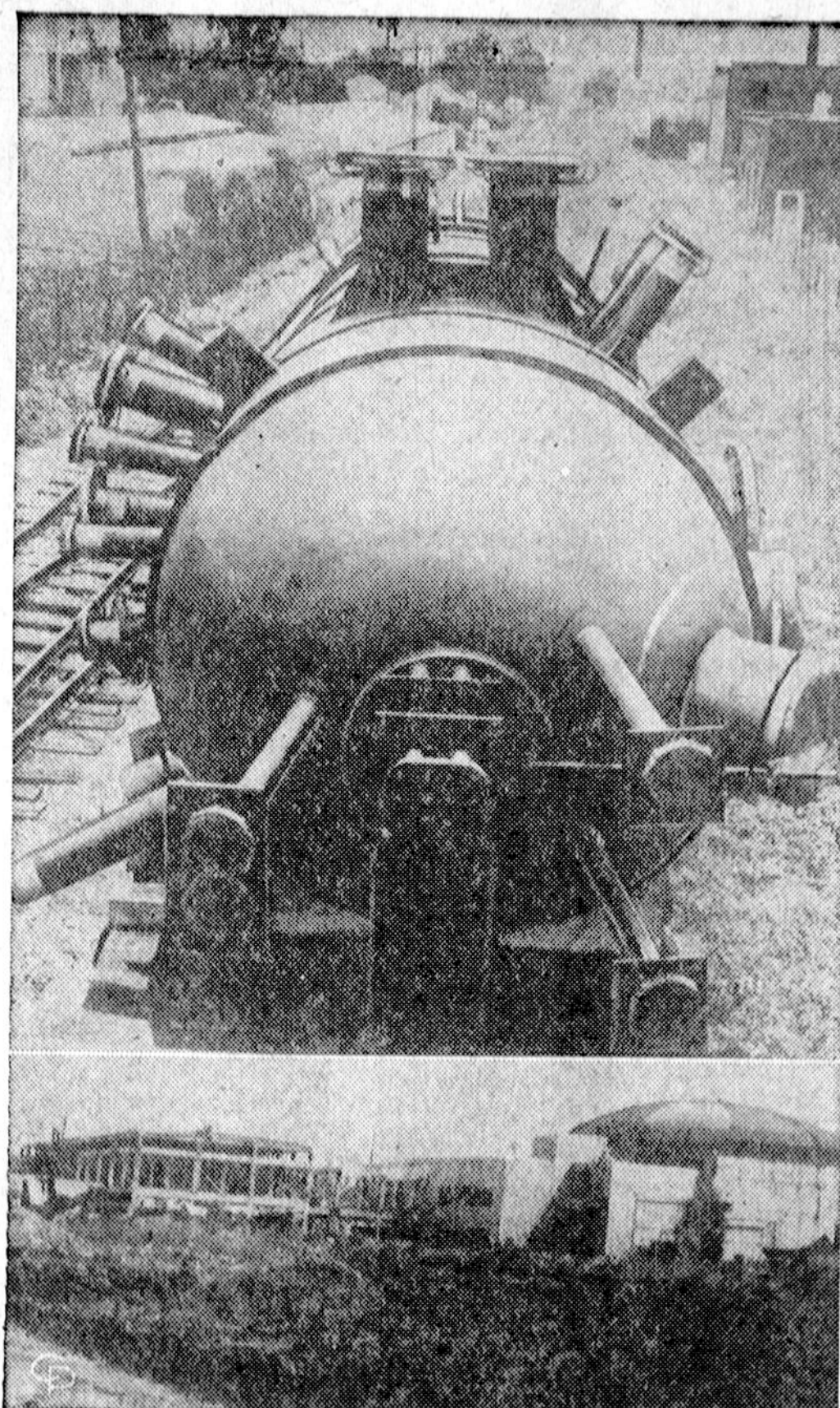
70 tonų spaudimo tankas gabenamas į Plum Brook, O., statomą fabriką (apatinė nuotrauka), kuriame bus pradėti gaminti atomine jėga varomi lėktuvai.
