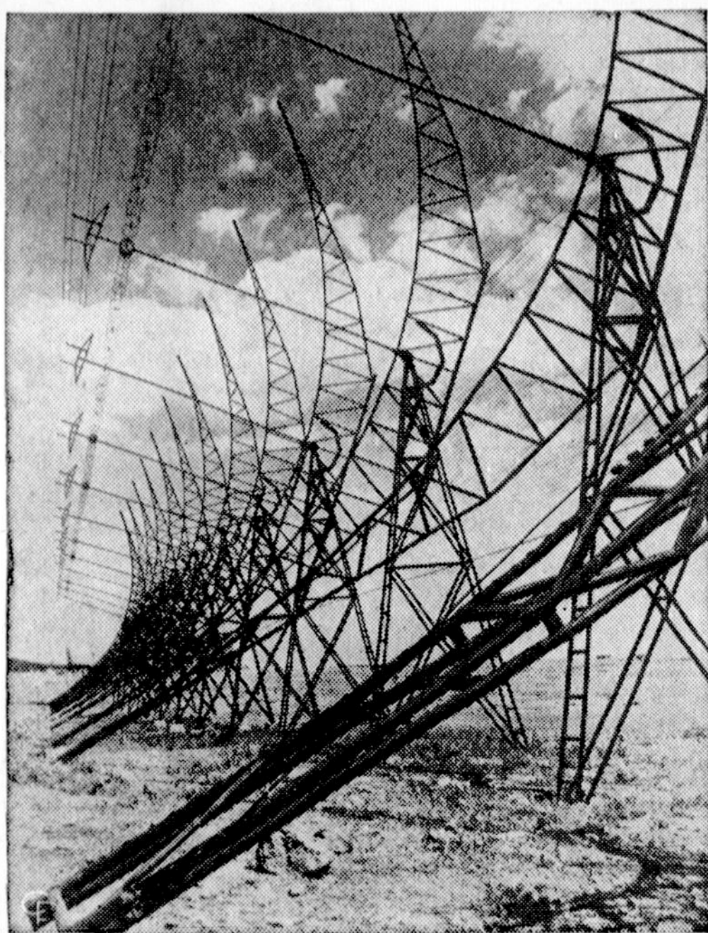
Dar nebaigtos sovietinio radijoteleskopo antenos astrofizinėje Biurakano observatorijoje. Radijoteleskopas bus naudojamas erdvės kūnų radiacijos šaltiniams ir tolimųjų žvaigždžių sistemoms stebėti.
