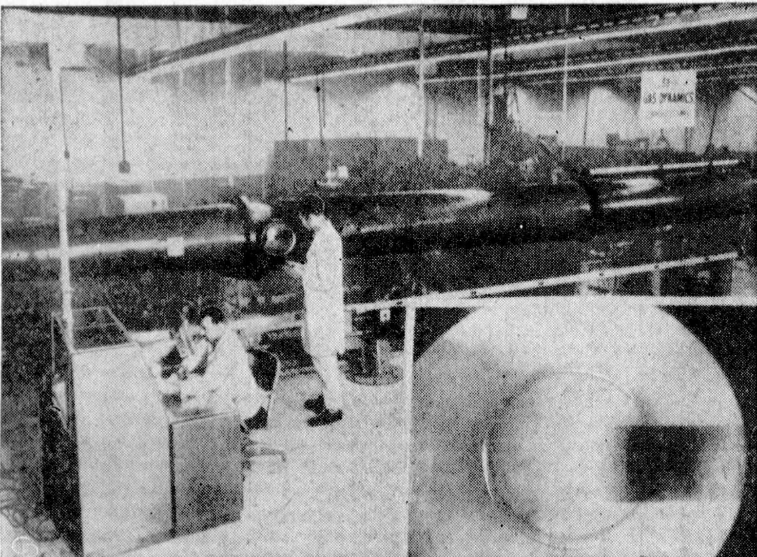
19 kartų už garsą greitesnis vėjo tunelis, kuriame tiriami naujų lėktuvų modeliai, Lockheed bendrovės laboratorijoje. Modelis stebimas pro specialų langelį vamzdyje.
