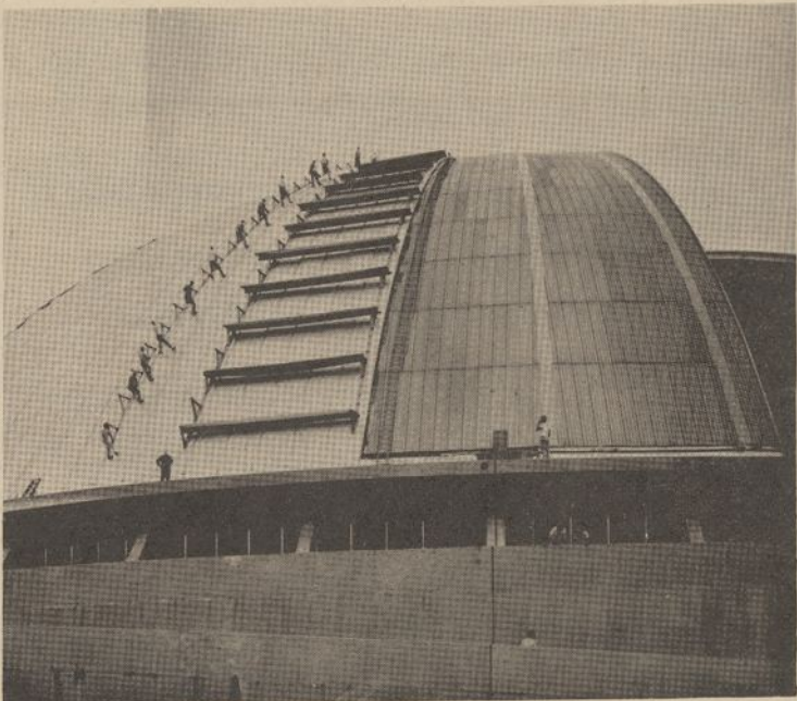
Pittsburgho miesto auditorijos stogas dengiamas iš nerūdijančio plieno ir stiklo. Mygtuko paspaudimu šis 136 pėdų aukščio ir 415 pėdų pločio stogas lengvai atsідarys. Tai pirmas tokios rūšies pastatas.
