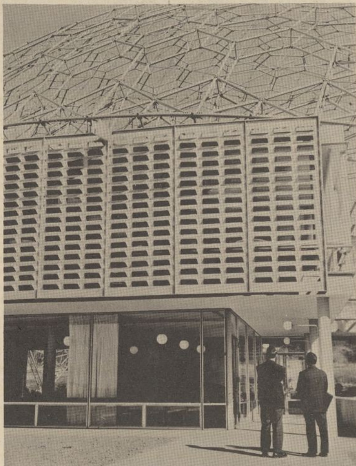
Statant Amerikos Metalinės Statybos draugijos pastatą Novelty, Ohio, buvo naudojamas nerūdijančio plieno sietas, kuris per stiklines sienas kontroliuoja saulės spindulių kiekį.
