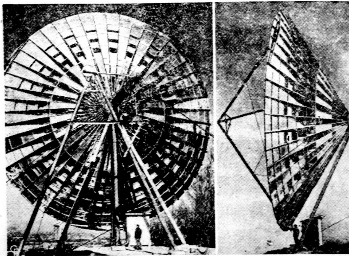
Prie Holmdel, N. J., bandymo tikslams patatyta didžiausia pasaulyje antena. Ji galėsianti be tarpinių stočių tiesiai per erdvę pagauti telefono ir televizijos signalus net iš 200 mylių atstumo. Kairėje antenos užpakalis, dešinėje ji matoma iš šono.
