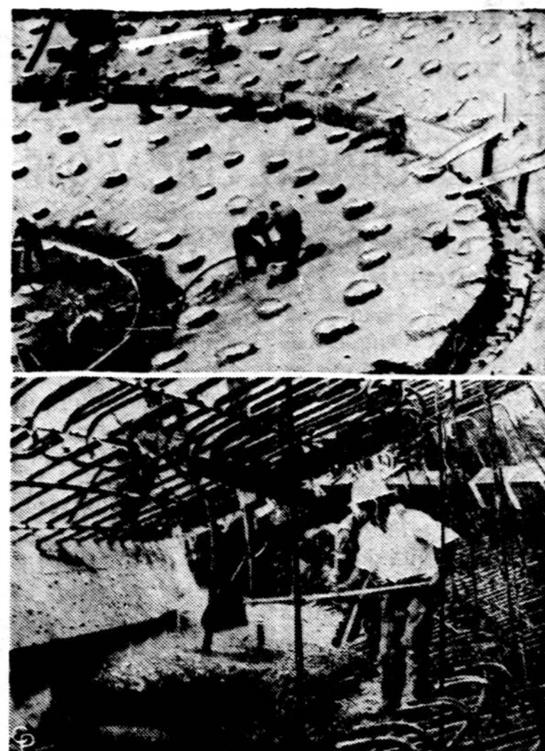
Italija stato atominę elektrinę netoli Neapolio. Viršuje matyti rūsių stulpai, o apačioje darbininkai traukia apie naujai įrengiamą atominį reaktorių. Nauja elektrinė gamins 150.000 kilovatų elektros energijos.
