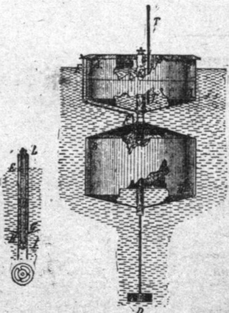
Evaporometras Luboslavskio.
