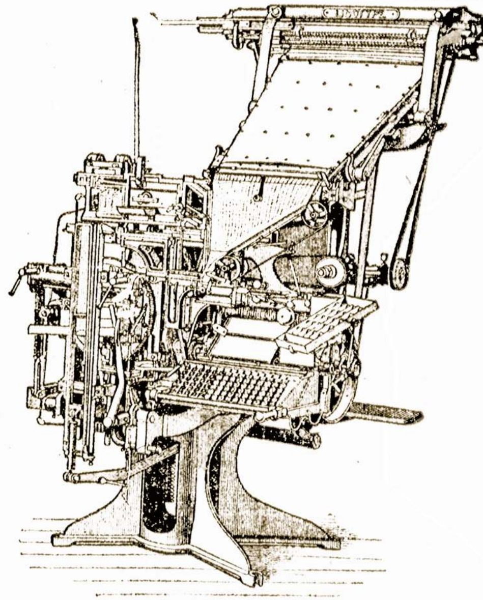
Linotype Model 5.—Raidžių Statomoji Mašina.
