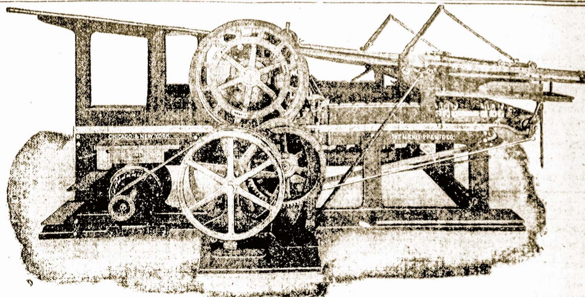
Miehle Presas.—Spausdinimui knygų, konstitucijų, cirkulių, bizniškų programų, langinių plakatų ir kitų didelių spaudinių.
