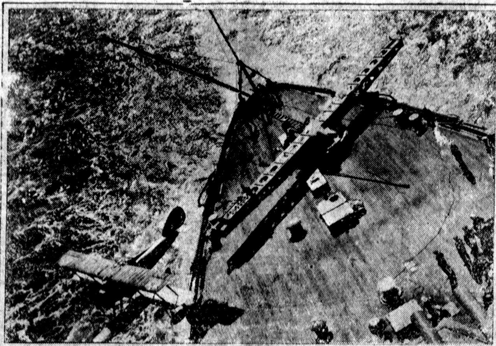
Fotografija nuimta San Diego uoste, nuleidžiant katapulto pagalba aerohidroplaną nuo Jungt. Valstijų karo laivo California prieš išvykstant į laivyno manevrus Havajų vandens
