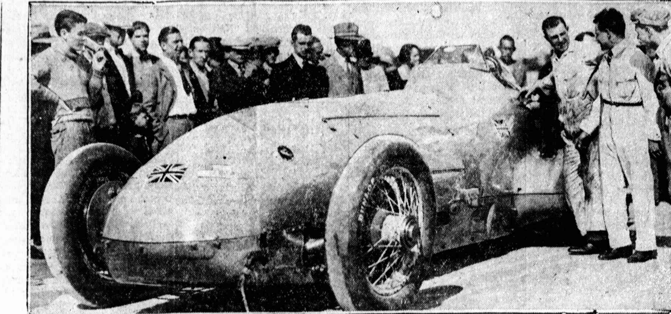
Greifiausias automobilis pasauly. Su juo anglų kapt. Malcolm padarė Dayton Beach, Fla., pajury virš 207 mylių į valandą — pasaulinį greitumo rekordą. Automobilis yra Anglijos konstru keijos.
