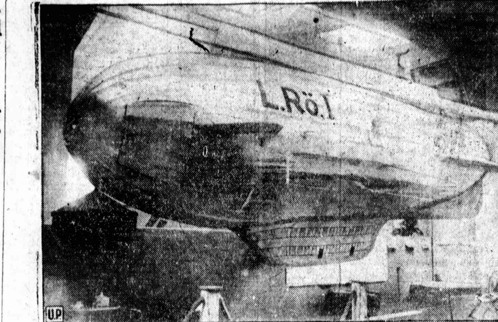
Derizablis L-Rö-1, kuris neužligo bus užbaigtas. Jis yra dirbamas Kaiserdamme (Vokietijoje). Jis kainuos $1,500,000 ir iš Vokietijos į New Yorką galės atskristi per 36 valandas. Tai bus didžiausias derizablis, kuris galės vežti 200 pasažierių.
