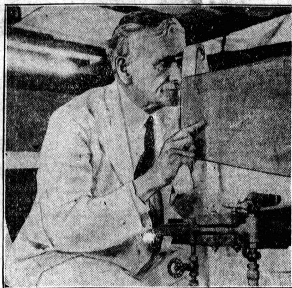
Chicago universiteto fizikos profesorius Dr. Albert A. Michelson, už savo mokslinius darbus laimėjęs Nobelio dovaną, pagelba savo paties pagaminto instrumento tyria šviesos greitumą. Jis galutinai nustatė, kad šviesa keliauja greičiu 299.796 kilometrų į sekundą.
