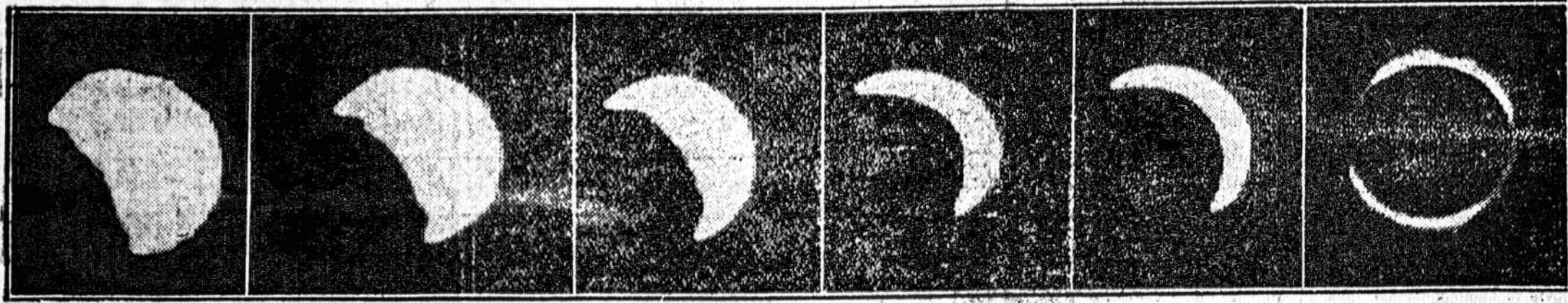
Fryeburg, Me. — Saulės užtemimo paveikslų serija, kuri buvo nuimta iš lėktuvo rugpjūčio 31 dieną.
