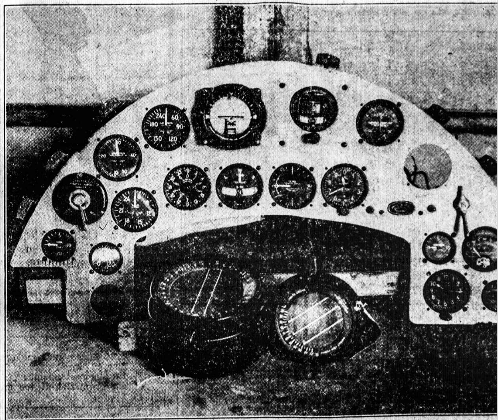
"Lituanicos II" didžioji instrumentų lenta, su dalimi navigacinių ir motoro instu
